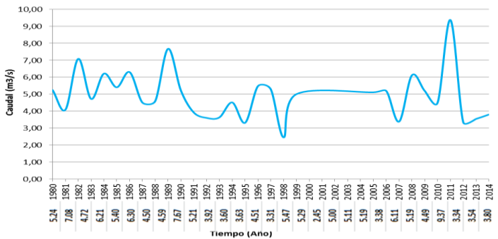
Caudal Medio Anual Estación El Guayabo IDEAM y RIMAC
