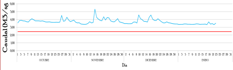
CAUDAL PROMEDIO DIARIO DEL GUAYABO
